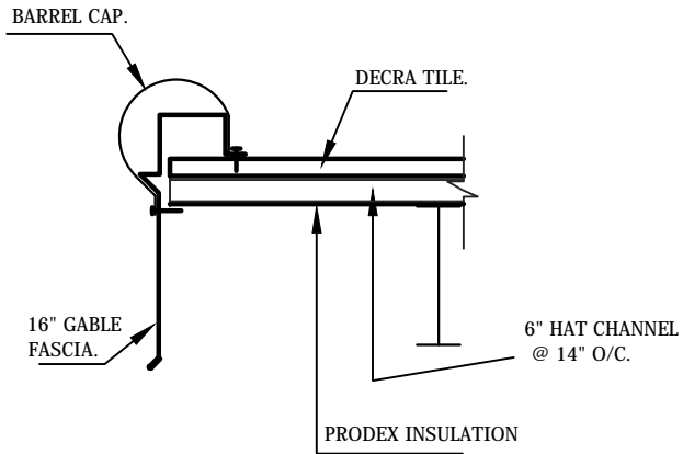
○ DECRA-GABLE FASCIA DETAIL Scale:
